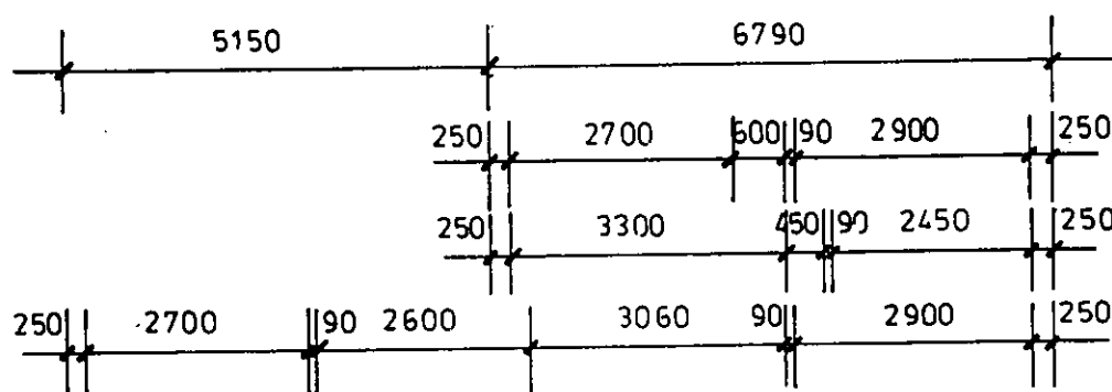
N.E. ELEVATION
