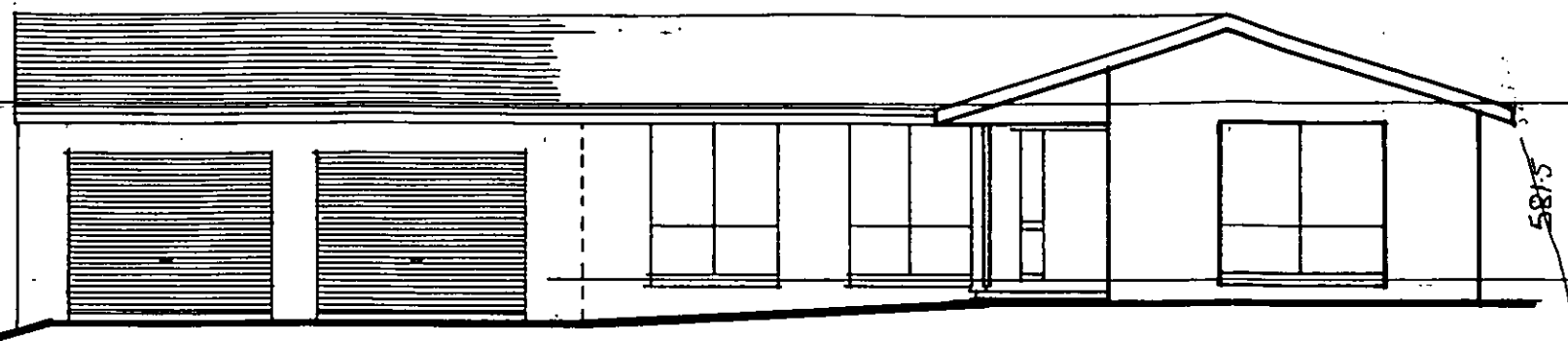
N.E. ELEVATION
