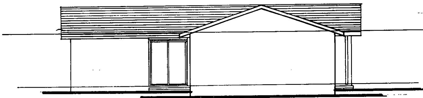
S.E. ELEVATION
