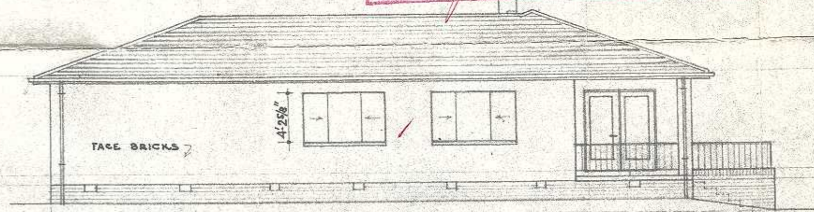
ELEVATION E
