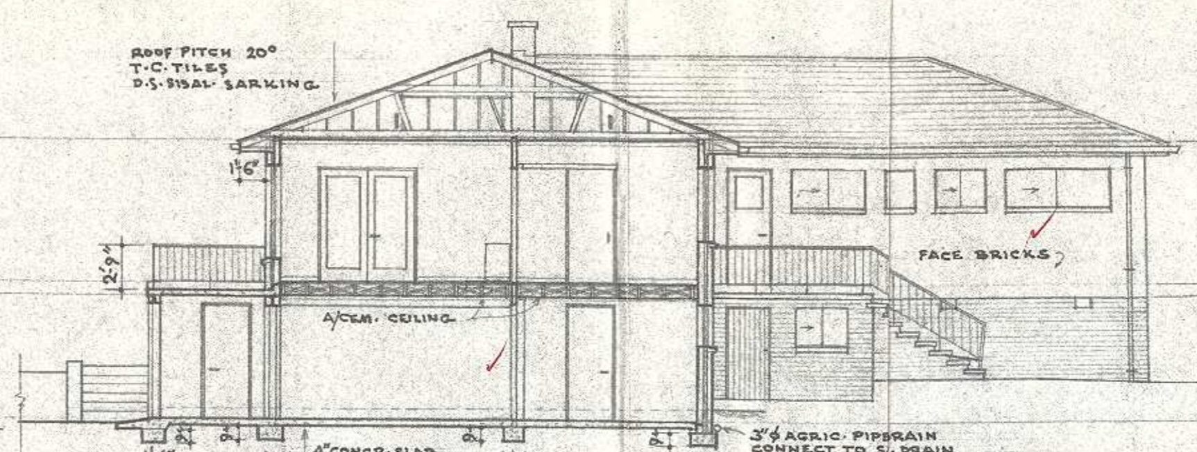
SECTION A-C
