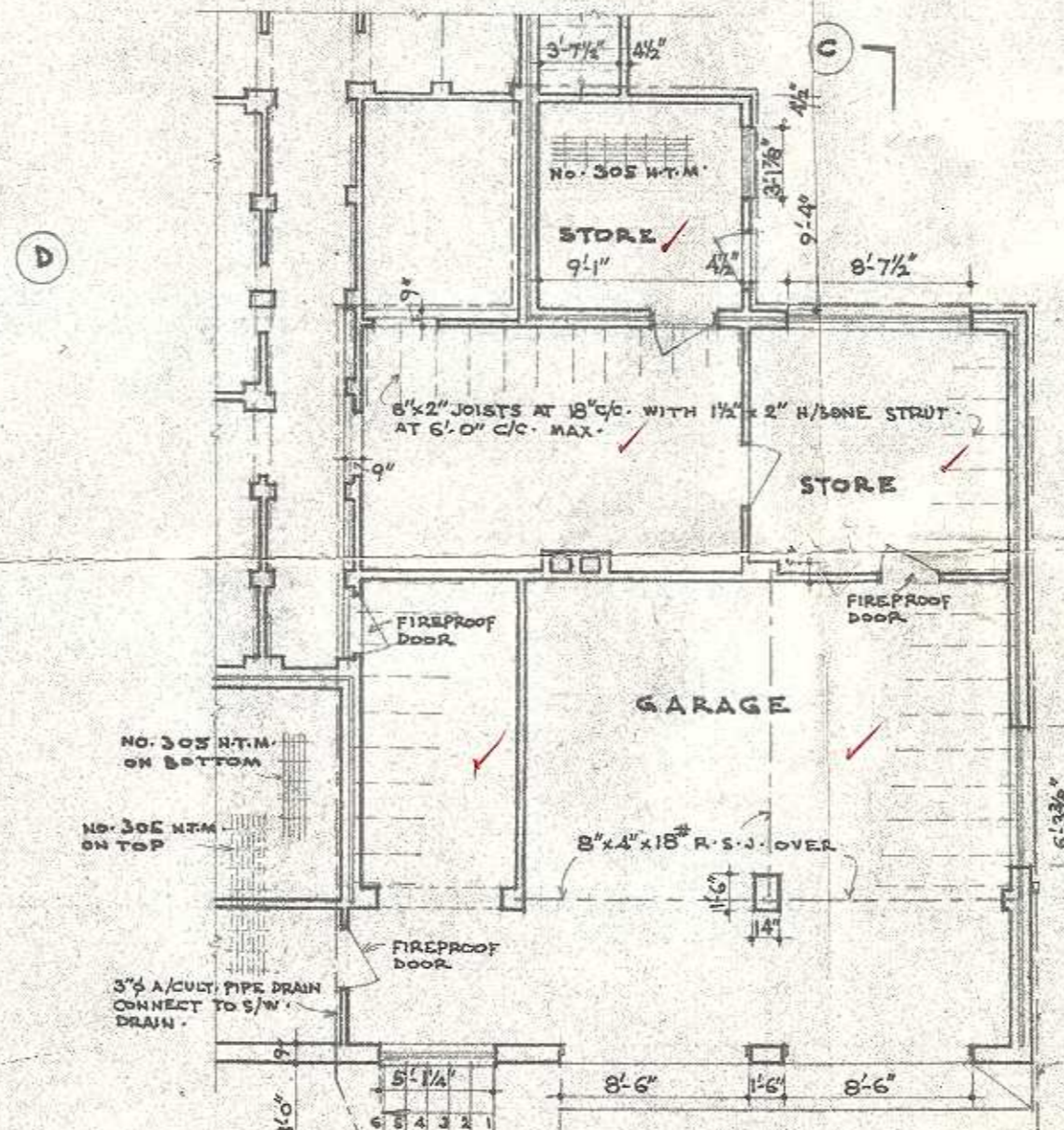
BASMENT PLAN SCALE: 1/8" = 1'-0"
