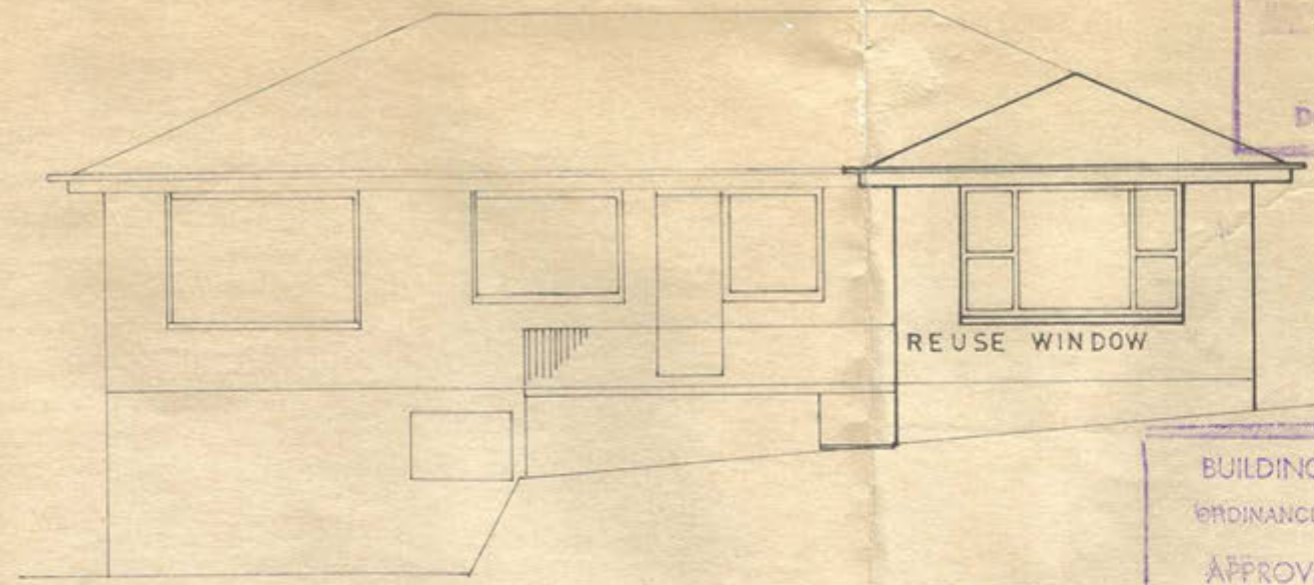
ELEVATION 1
