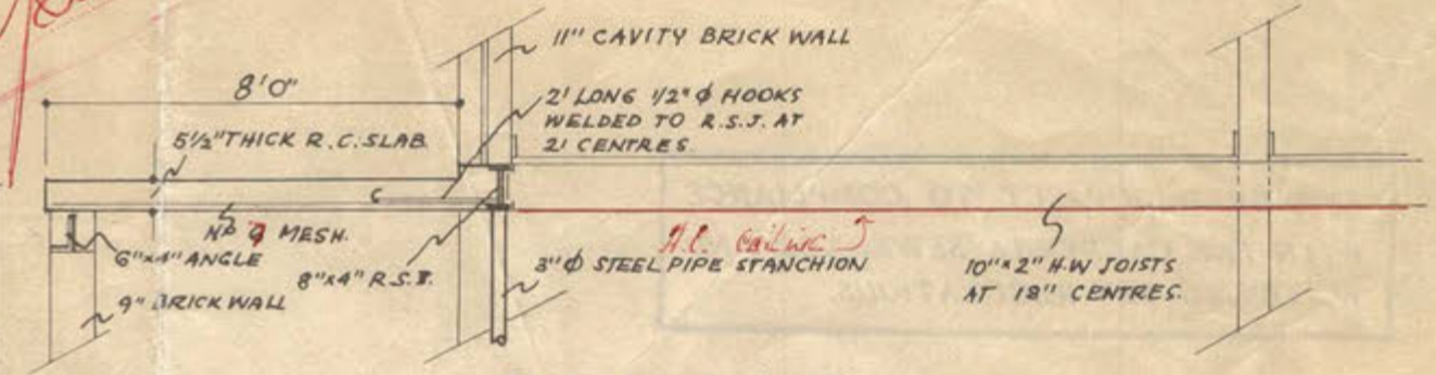
SECTION A-B
