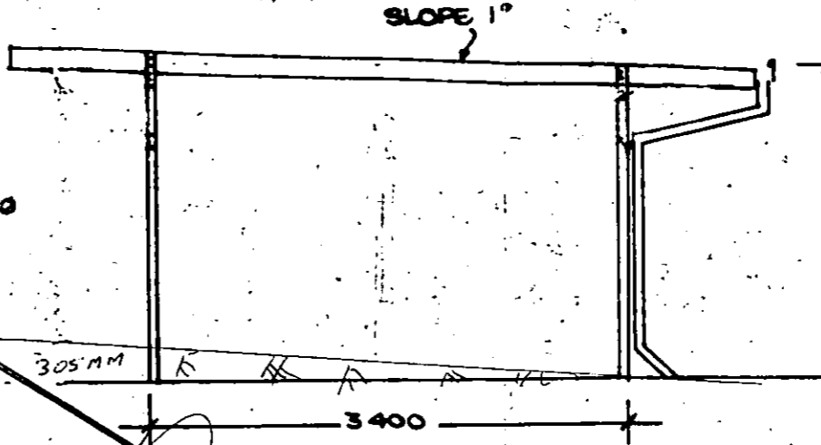
ELEVATION B
