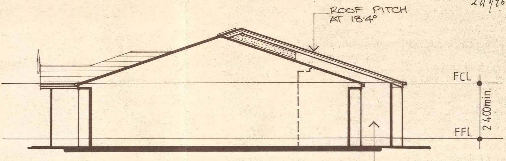
R.H. SIDE ELEVATION 1:100
