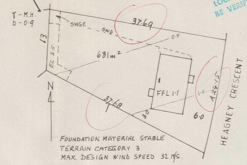
Site plan 1:500
