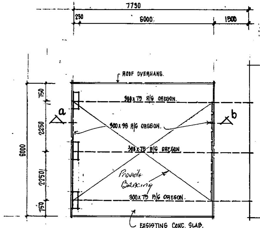
plan 1:100
