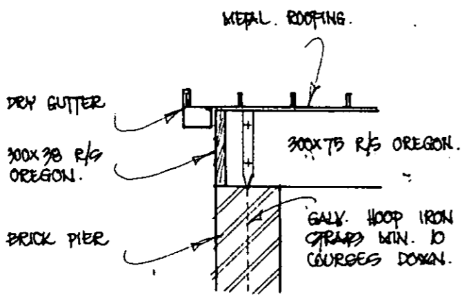
detail a-a 1:20
