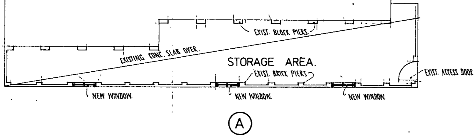
PLAN.
