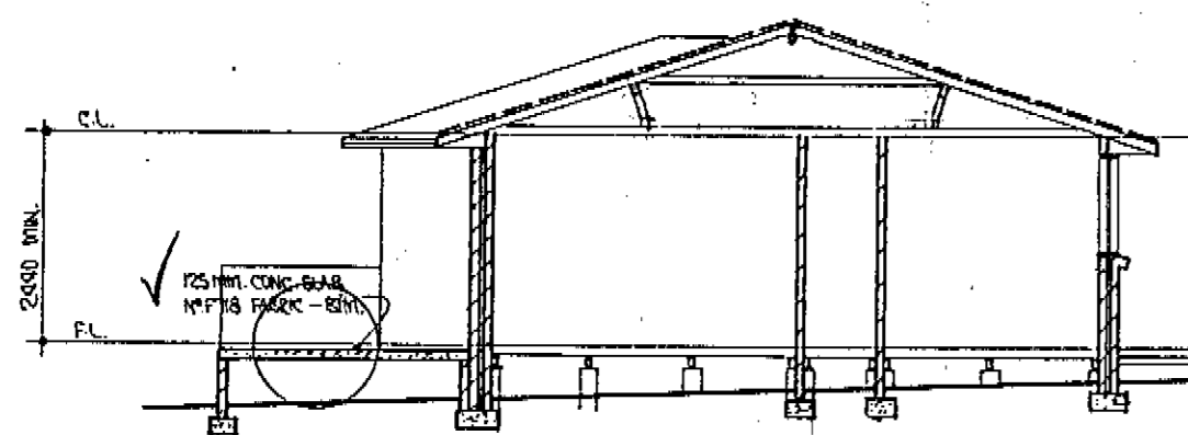
SECTION A-A.
