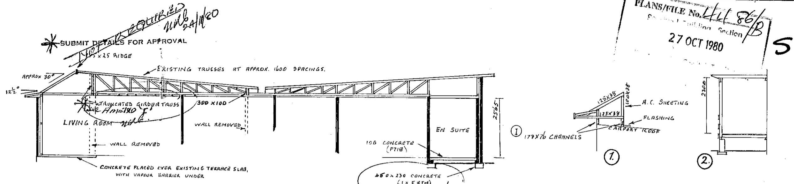
Section A-A
