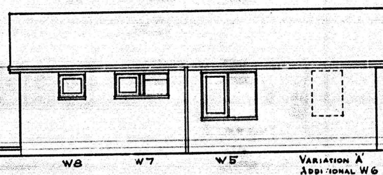
ELEVATION ②
