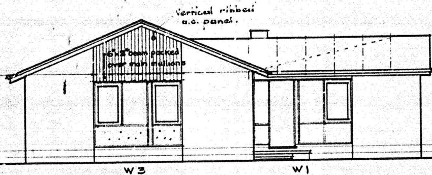
ELEVATION ①
