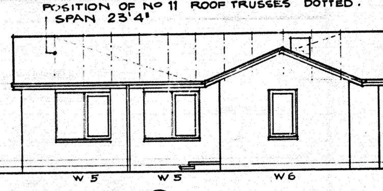
ELEVATION ④
