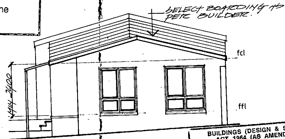
ELEVATION 1
