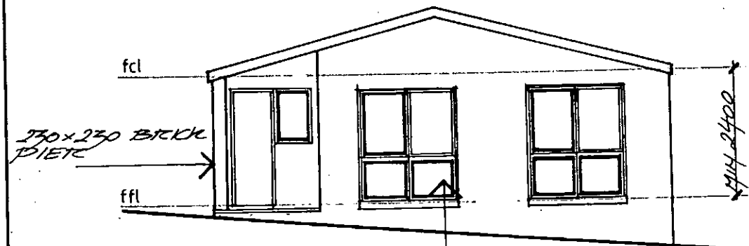
ELEVATION 3
